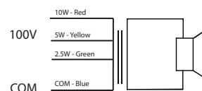
SP 10EN Circuit diagram
